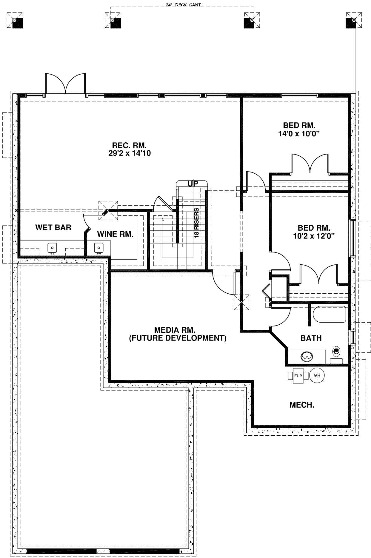
BASEMENT - 1223 SQ.FT.
